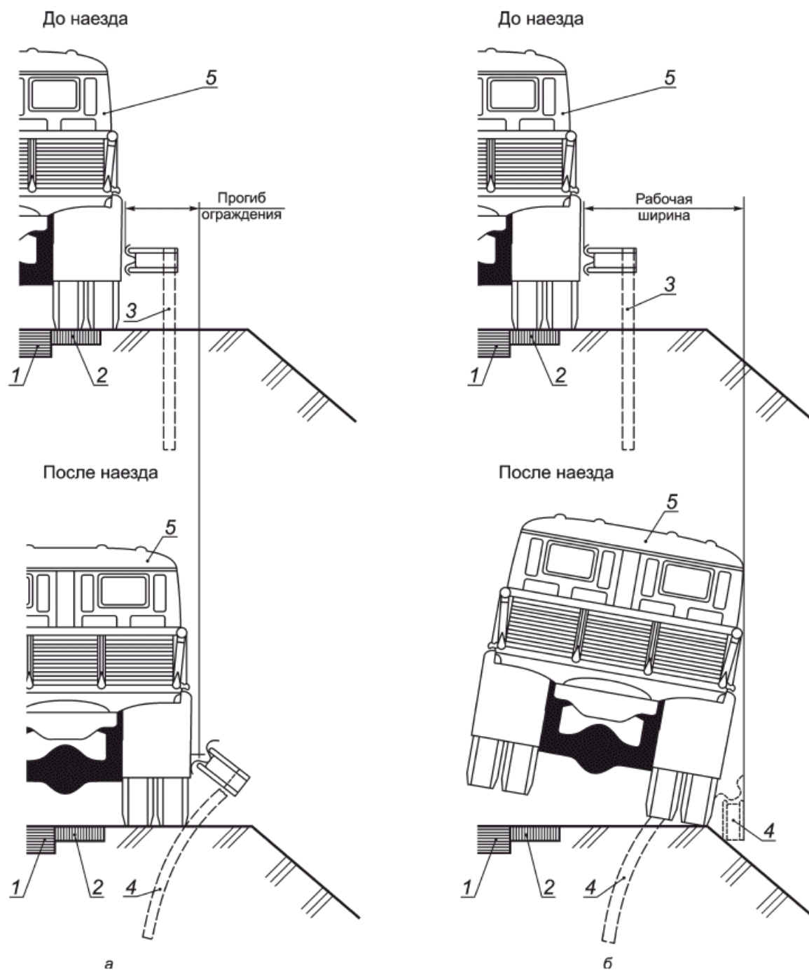
а - прогиб; б - рабочая ширина дорожного ограждения 1 - проезжая часть; 2 - укрепительная полоса; 3 - недеформированное ограждение; 4 - деформированное ограждение; 5 - транспортное средство
