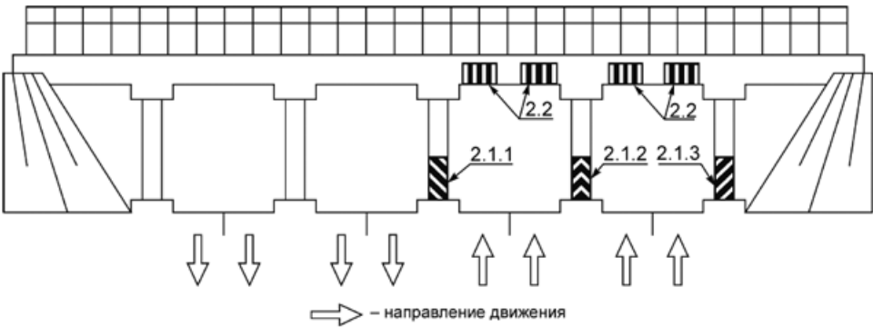
Рисунок В.22 - Пример нанесения разметки 2.1 и 2.2
