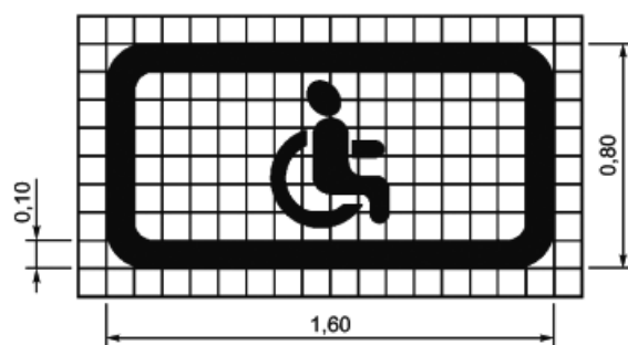
Рисунок Б.16 - Размеры разметки 1.24.3
