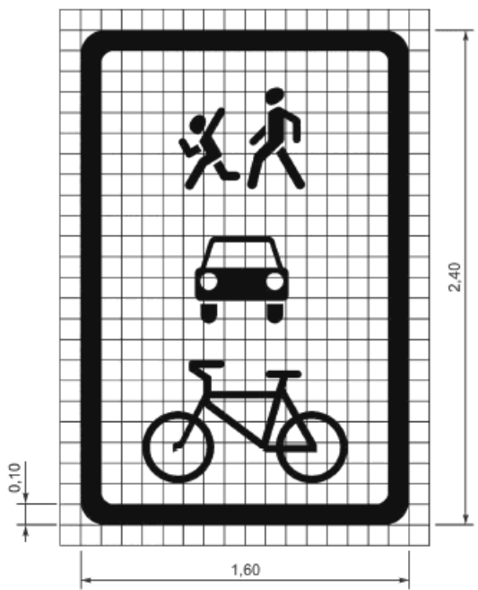
Рисунок Б.19* - Размеры разметки 1.24.6
