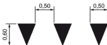
Рисунок Б.1 - Размеры разметки 1.13
