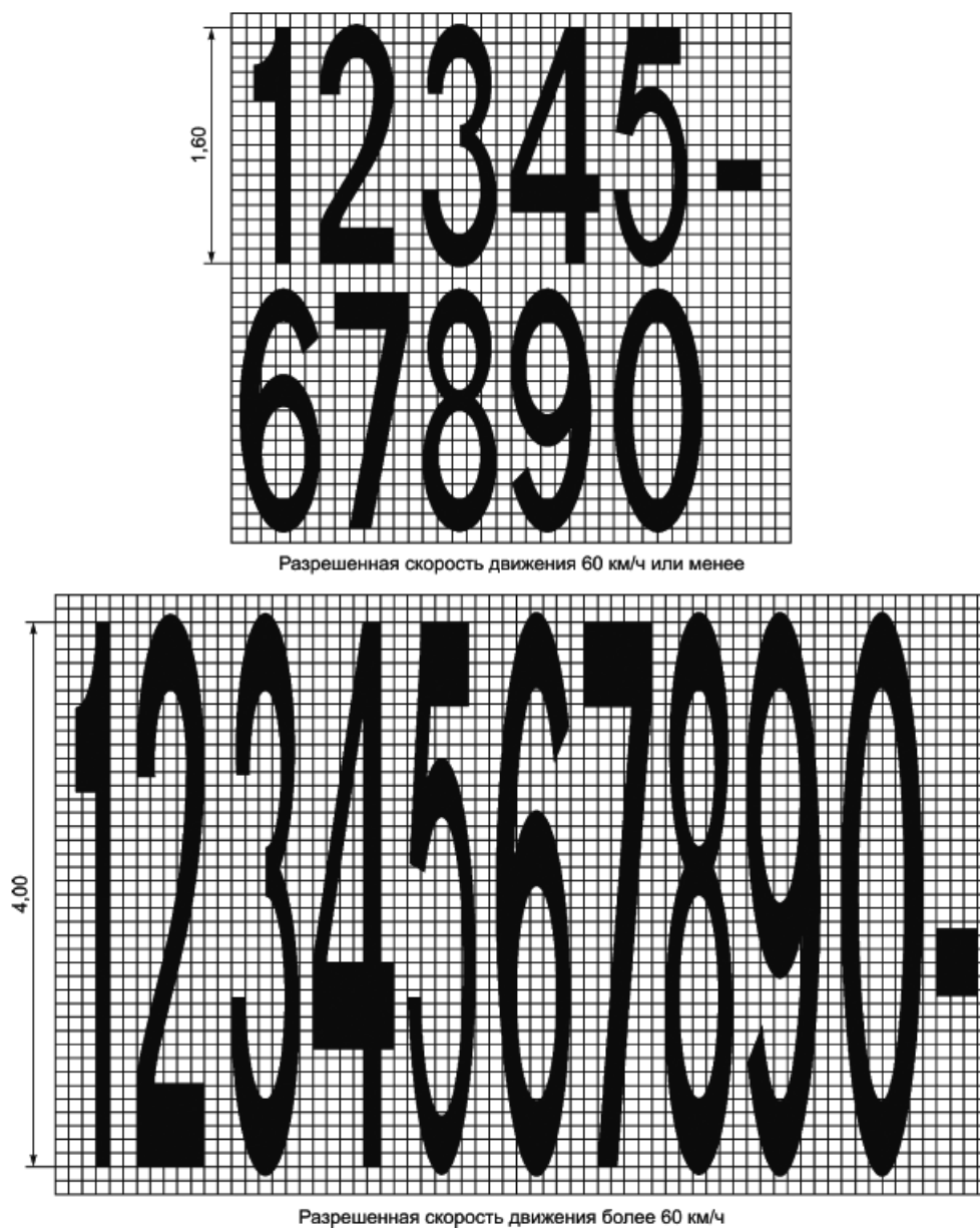
Рисунок Б.9 - Расположение и размеры цифр разметки типа 1.22
