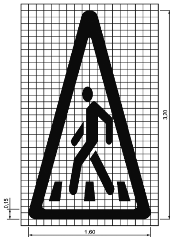
Рисунок Б.14 - Размеры разметки 1.24.1
