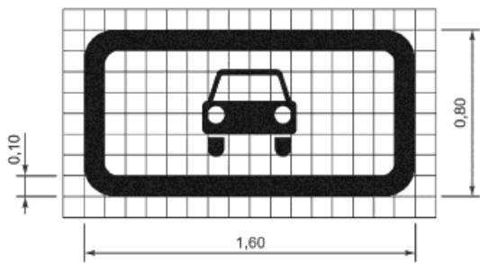
Рисунок Б.20* - Размеры разметки 1.24.7
