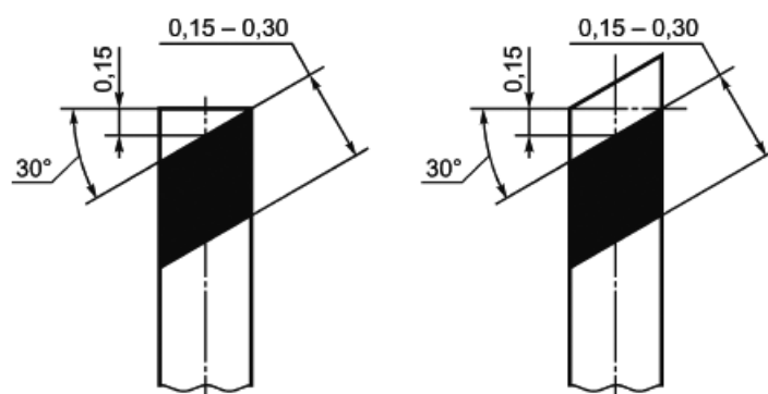
Рисунок Г.2 - Размеры разметки 2.4
