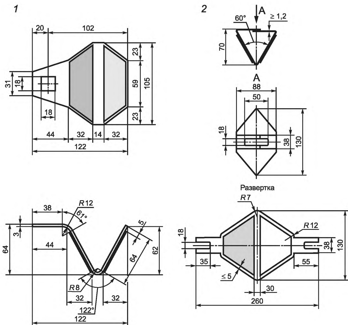
Рисунок Б.4 — Световозвращатель типа КД4
