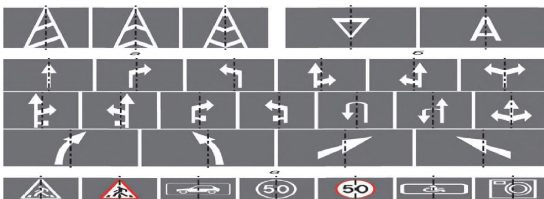
а – для горизонтальной разметки в виде наклонных полос (включая ломанные), ограниченных сплошными одиночными линиями; б – для горизонтальной разметки в виде равнобедренного треугольника, обращенного вершиной к водителю, не окрашенного внутри и для горизонтальной разметки в виде изображения буквы «А»; в – для горизонтальной разметки в виде изображения дорожного знака Рисунок 2 – Схема расположения осей горизонтальной разметки
