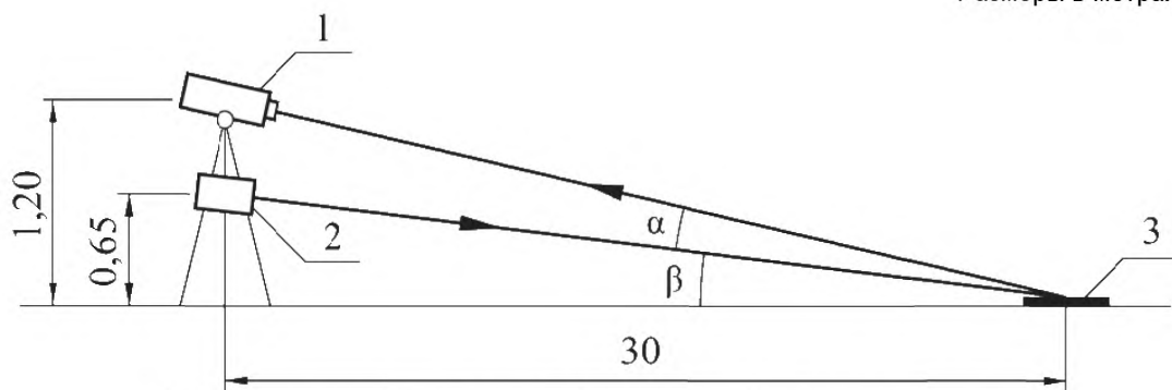
1 – фотоприемник; 2 – стандартный прожекторный источник света типа А по ГОСТ 7721, 3 – дорожная разметка
