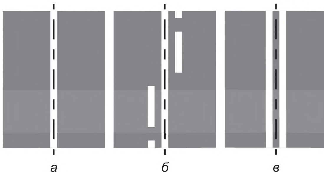
а – для горизонтальной разметки в виде сплошных и прерывистых одиночных линий; б – для горизонтальной разметки в виде сочетания сплошной одиночной линии и прерывистой одиночной линии с соотношением длины штриха к расстоянию между штрихами, равному 3:1; в – для горизонтальной разметки в виде двойной сплошной или прерывистой линии Рисунок 1 – Схема расположения осей линий горизонтальной разметки, наносимых вдоль оси автомобильной дороги
