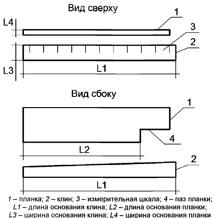
Рисунок 9 – Схема высоотомера для определения высоты выступающей горизонтальной дорожной разметки над поверхностью, на которую она нанесена
