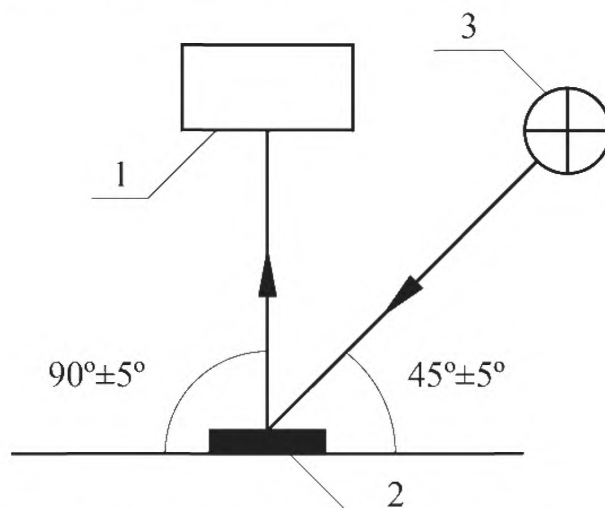
Рисунок 10 – Условия измерения координат цветности и коэффициента яркости
