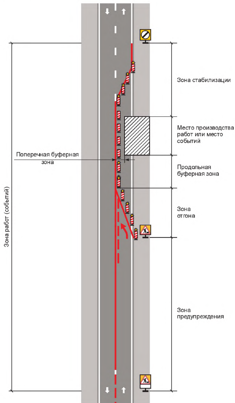
Рисунок А.1 — Схема зоны работ (событий), вызвавших необходимость временного изменения организации дорожного движения на автомобильной дороге
